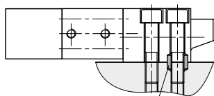
Zubehör: Bohrbuchsen
